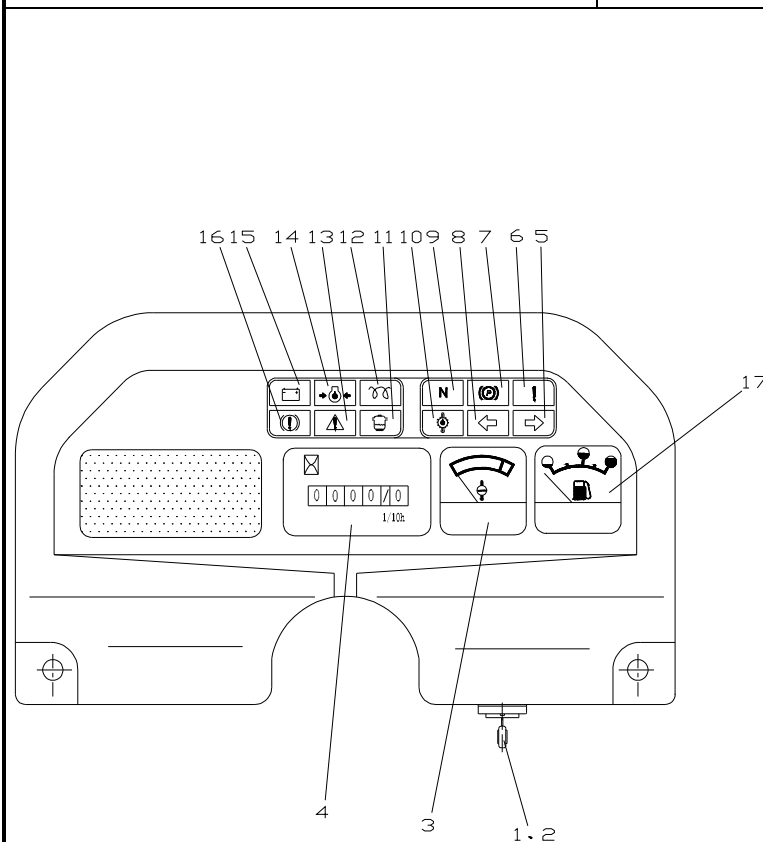
图XI 仪表板总成 (感知系统) Fig.XI Instrument assy (OPS System)
