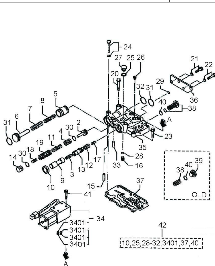
图 36 控制阀 Fig.36 Control valve
