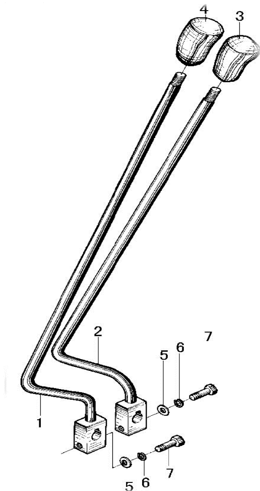
图 16 换挡操纵总成 Fig. 16 Change over control assy
