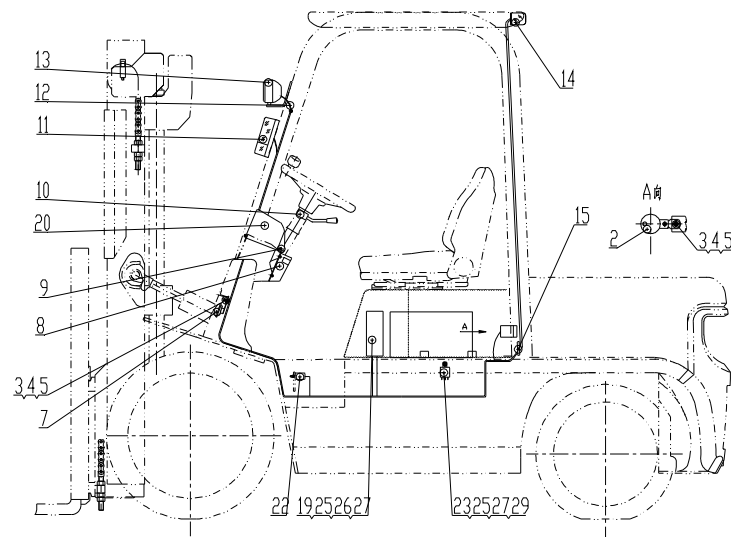
图 6-1 电气系统 Fig.6-1 Electrical system
