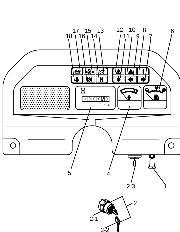
图 12-A 仪表板总成 Fig.12-A Instrument assy
