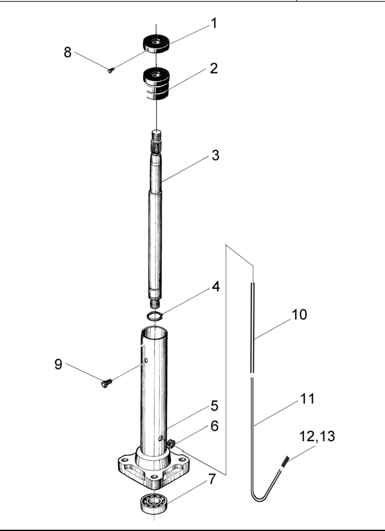
图6 转向管装置 Fig. 6 Steering pipe device
