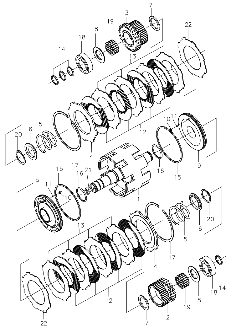
图 27 液力离合器(液力式) 中南 ZhongNan Fig.27 Hydraulic clutch(tor-con type)
