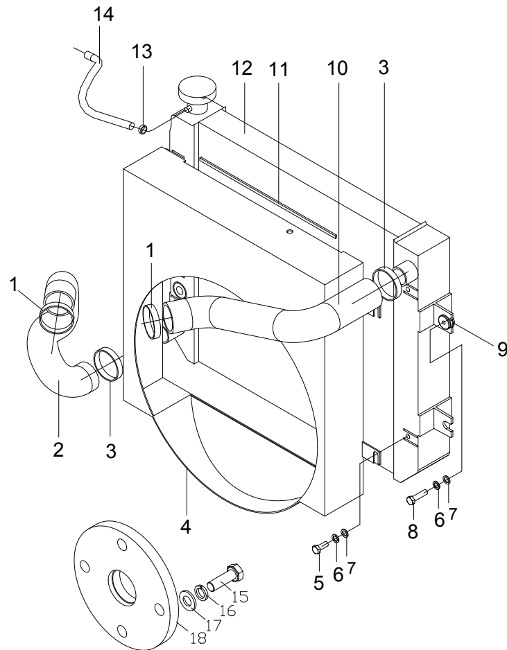
图 9-A 冷却系统 Fig.9-A Cooling system
