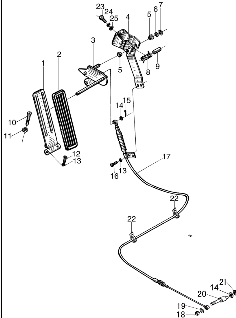
图 12 油门操纵总成 Fig. 12 Throttle control assy
