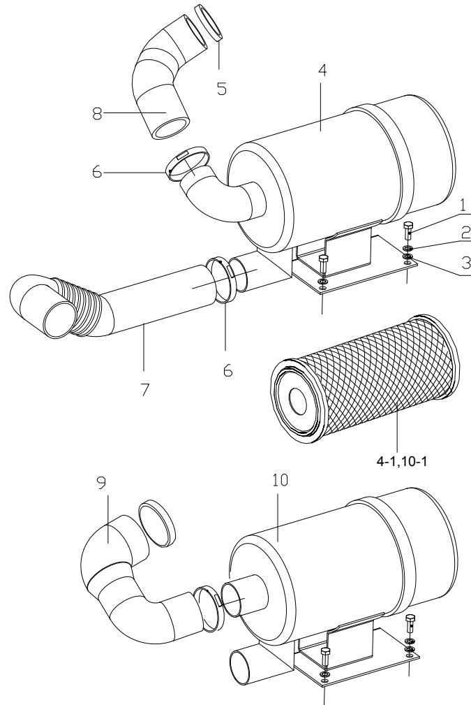
图 64 进气系统 Fig. 64 Air intake system
