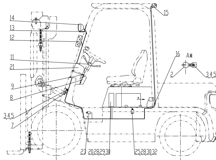
图 6-2 电气系统 Fig.6-2 Electrical system
