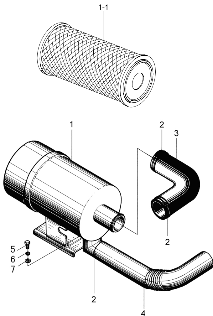
图3 进气系统 Fig.3 Air intake system
