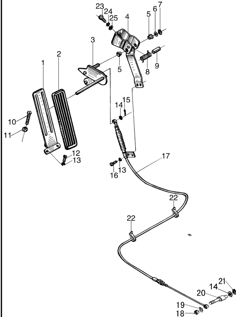
图 12 油门操纵总成 Fig. 12 Throttle control assy <2014-02-01
