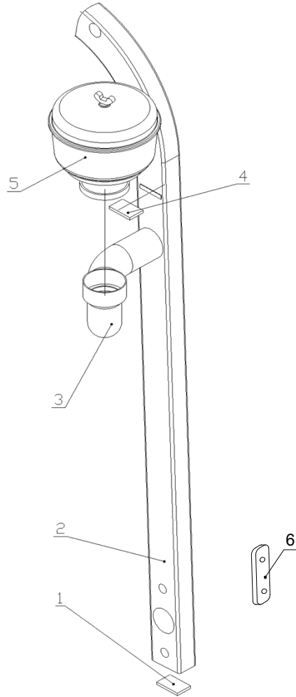
图 55 高位进气系统 Fig.55 High air intake system
