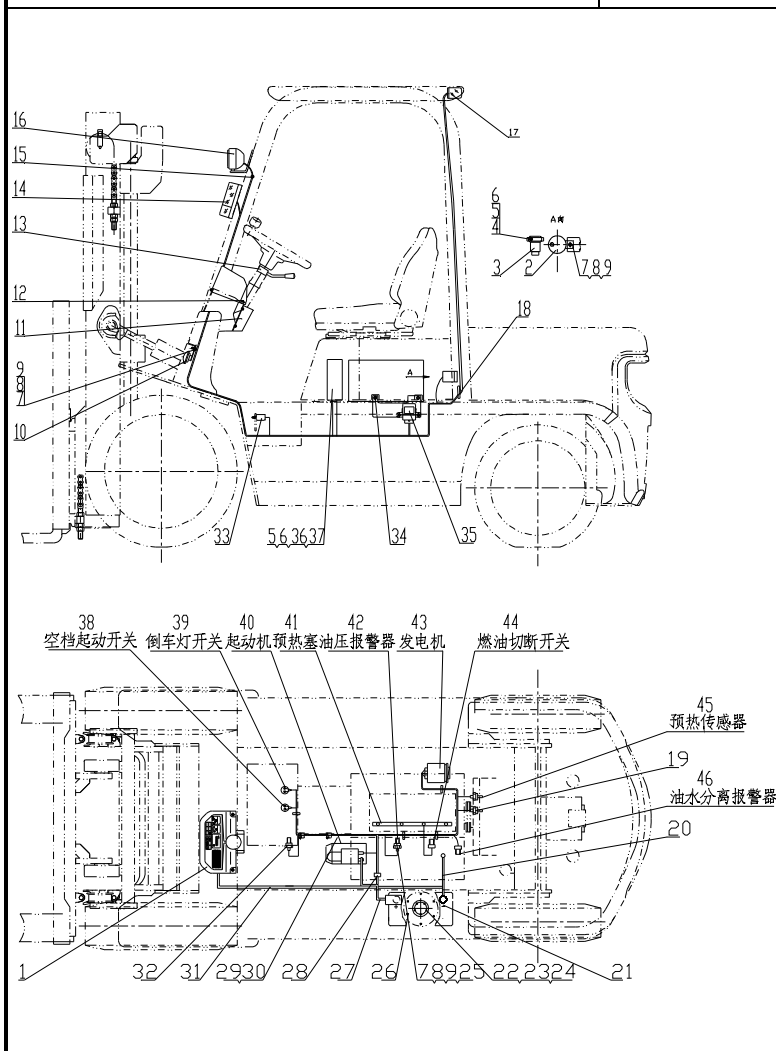
图 5 电气系统 Fig.5 Electrical system
