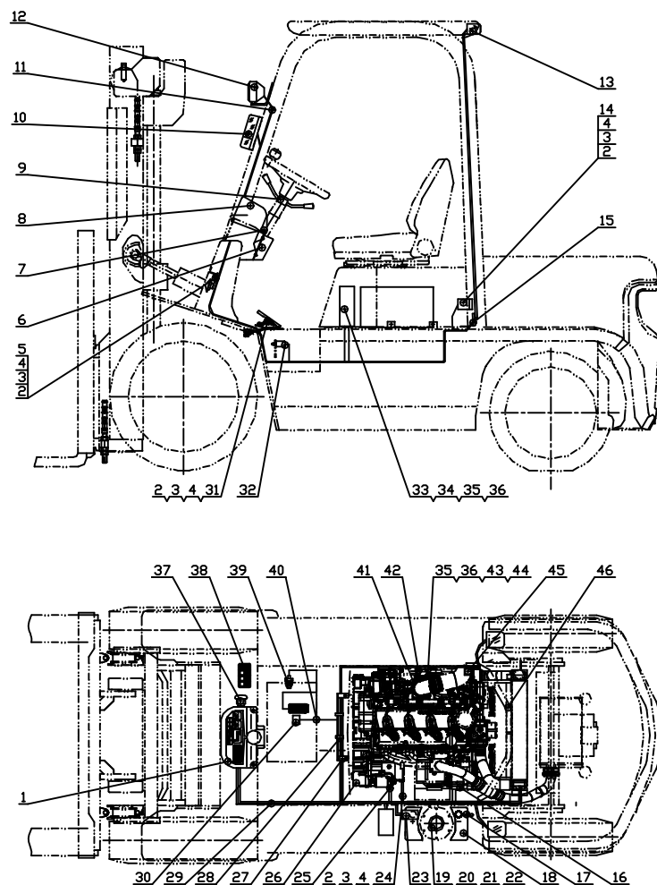
图 12 电气系统 Fig.12 Electrical system
