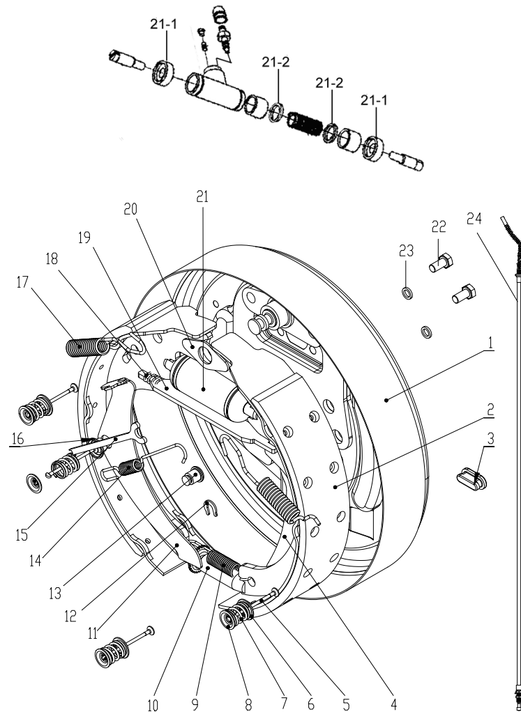
图 15-2 右制动器总成 Fig.15-2 Brake assy,RH
