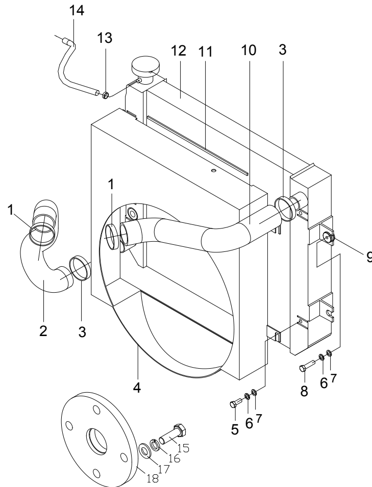
图 9-A 冷却系统 Fig.9-A Cooling system
