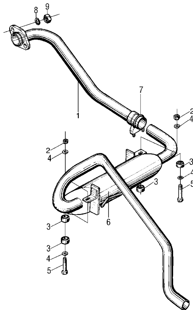
图 46 排气系统 Fig.46 Exhaust system
