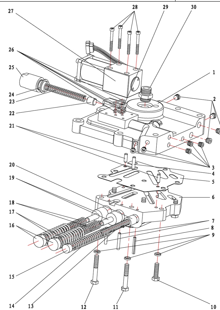
图 28 DCCT5 控制阀（液力式）中南 Fig.28 inching valve(tor-con type) ZhongNan
