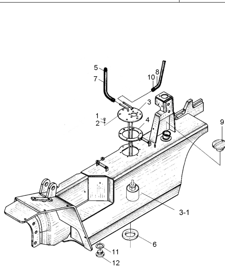
图 11 燃油系统 Fig. 11 Fuel system
