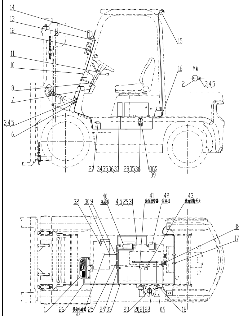
图 11 电气系统 Fig.11 Electrical system
