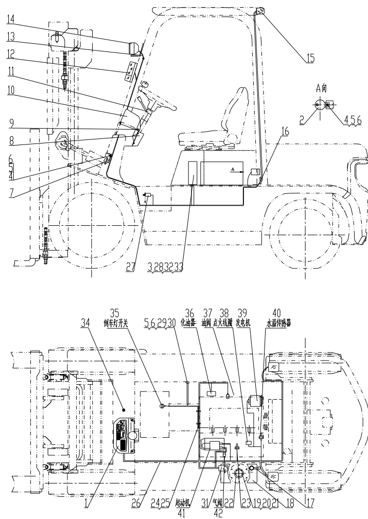
图 10-1 电气系统 Fig.10-1 Electrical system
