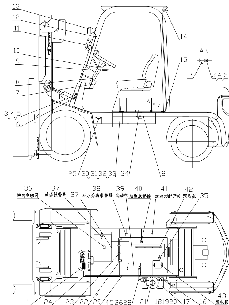
图 13 电气系统 Fig.13 Electrical system
