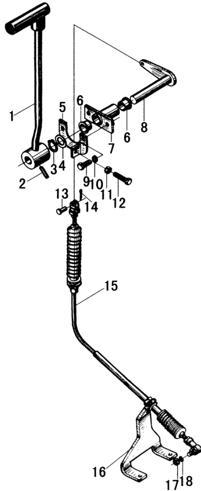
图 17 换档操纵总成 Fig. 17 Change over control assy
