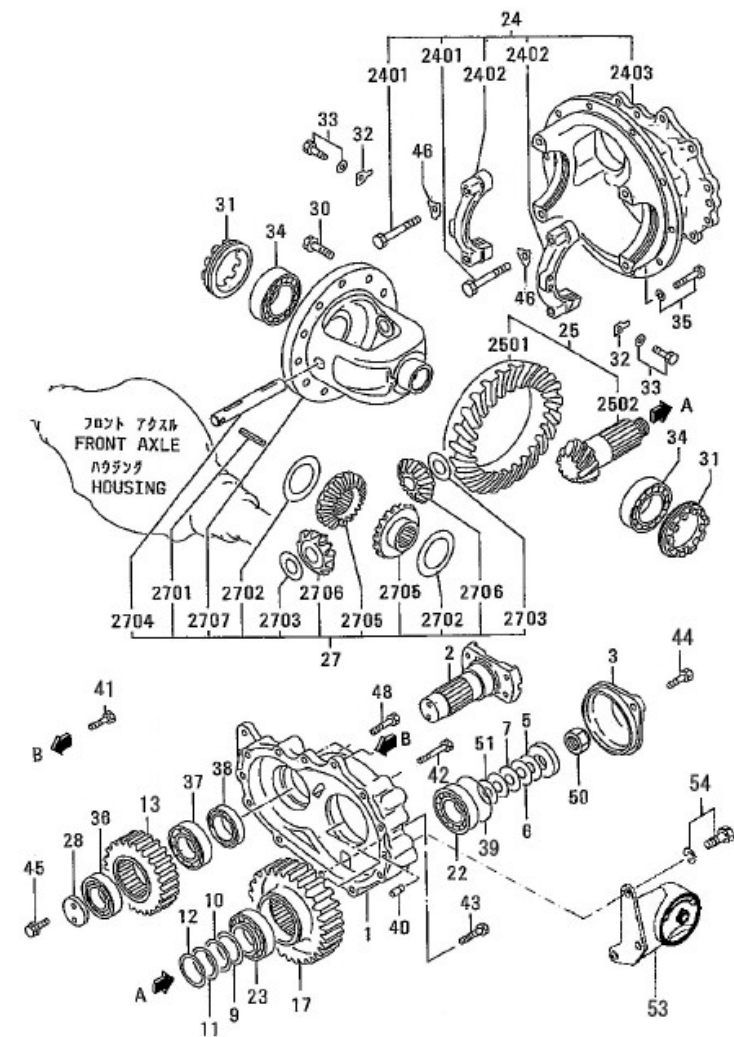
图 37 2.0-2.5t 主减速器·差速器总成 Fig.37 2.0-2.5t Reduction & Differential
