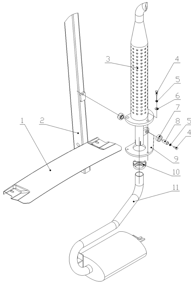
图 60 高位排气系统 Fig.60 High Exhaust system
