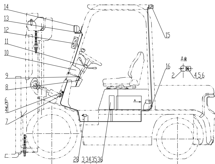
图 10-2 电气系统 Fig.10-2 Electrical system
