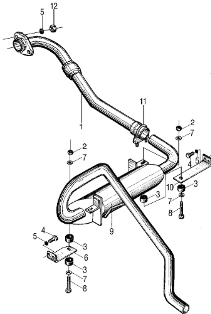
图 45 排气系统 Fig.45 Exhaust system
