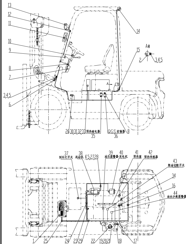
图 3-1 电气系统 Fig.3-1 Electrical system
