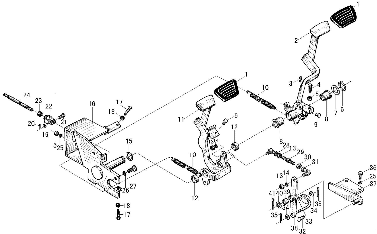
图 2 制动微动踏板总成 Fig. 2 Brake and inch pedal assy
