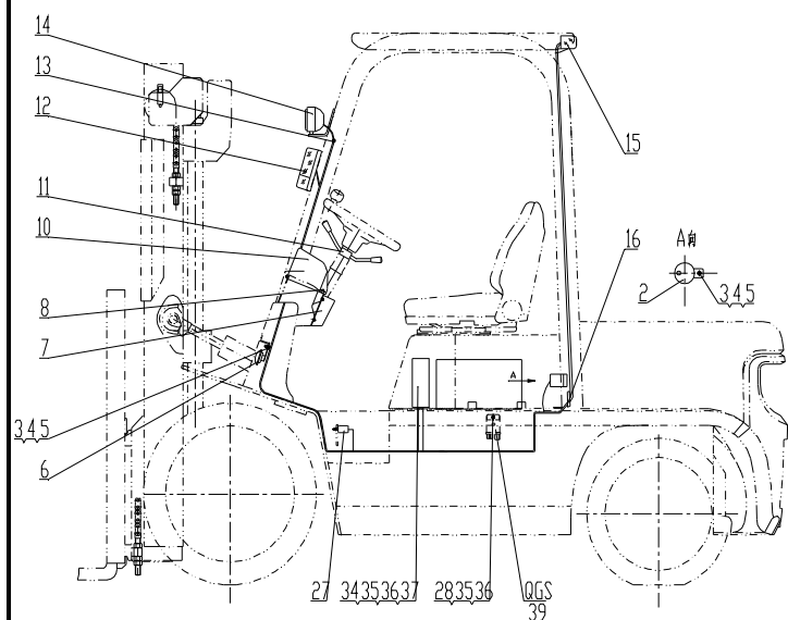
图 11 电气系统 Fig.11 Electrical system
