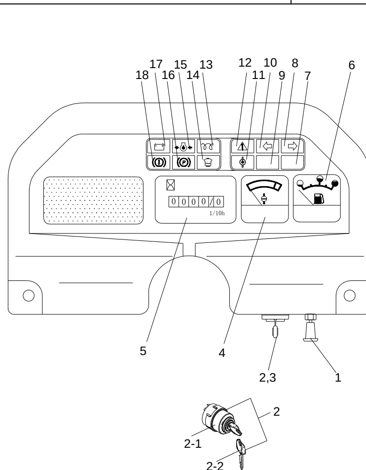
图 I 仪表板总成 Fig. I Instrument assy
