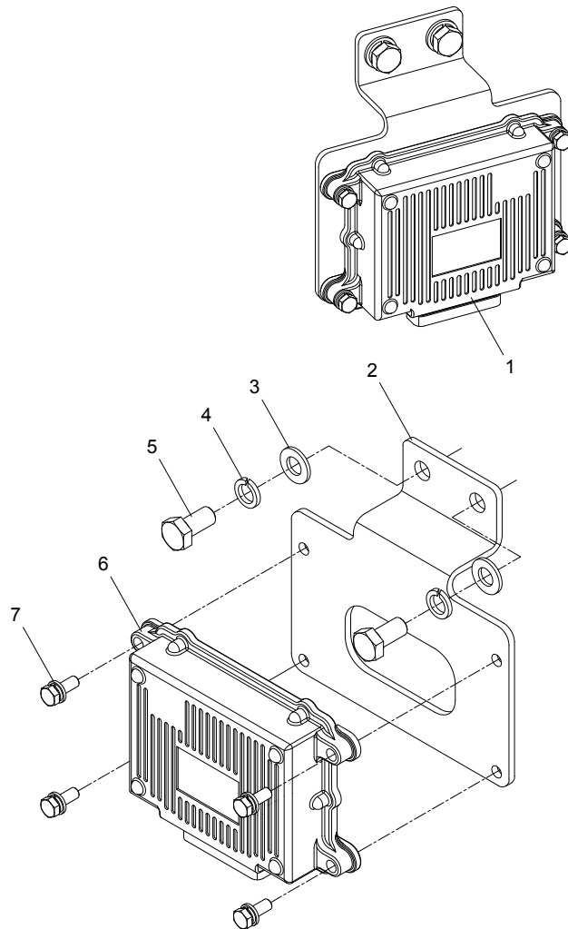
图 1-A 电控单元总成 Fig.1-A ECU assy
