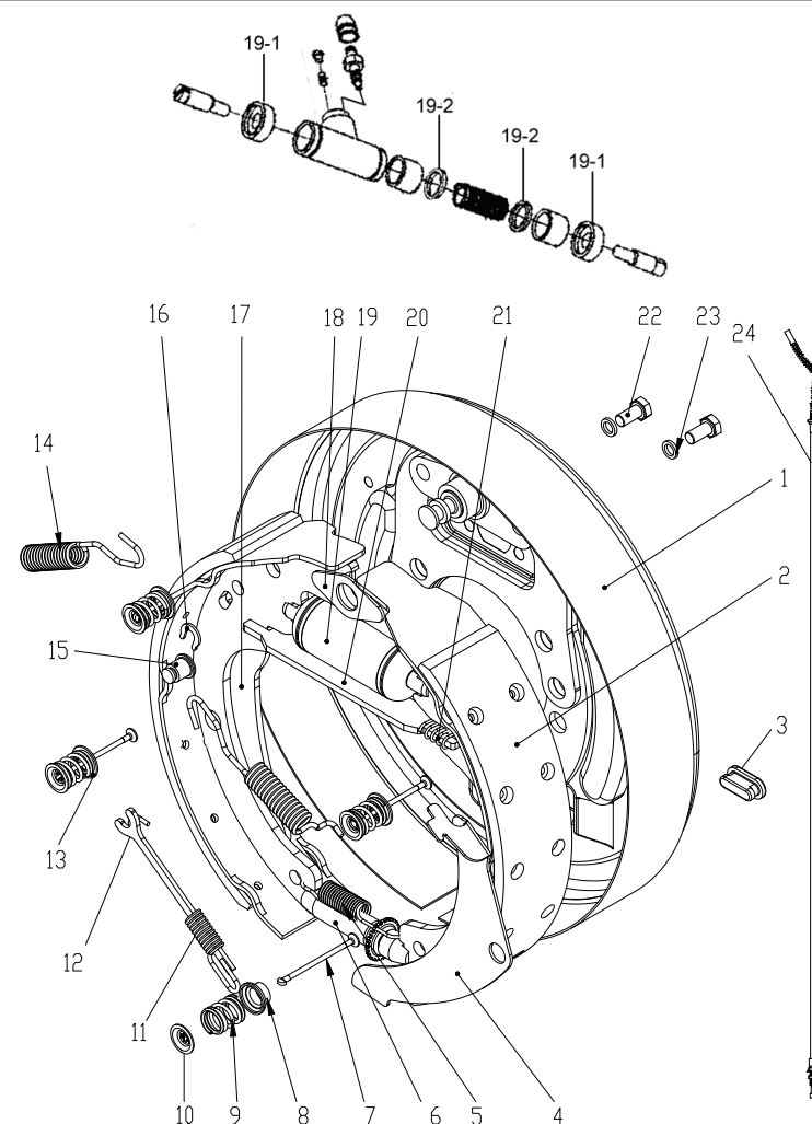
图 15-1 左制动器总成 Fig.15-1 Brake assy,LH
