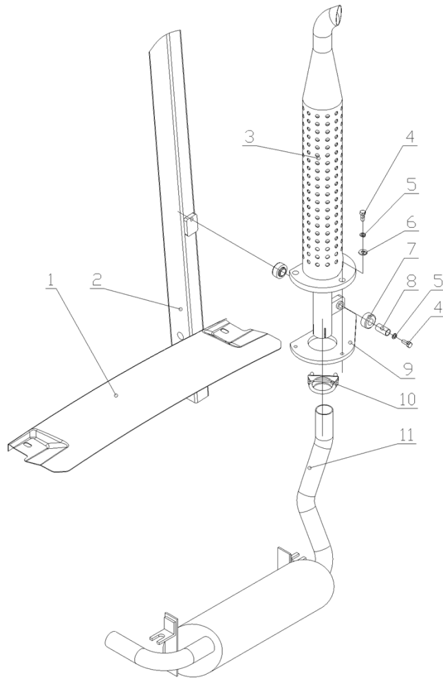
图 56 高位排气系统 Fig.56 High Exhaust system
